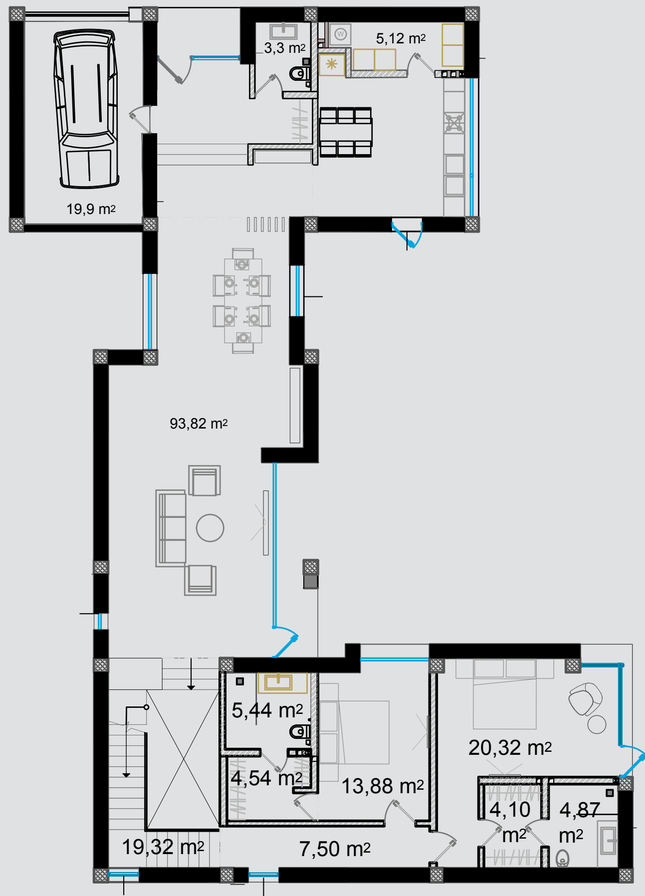
mərtəbə 1
